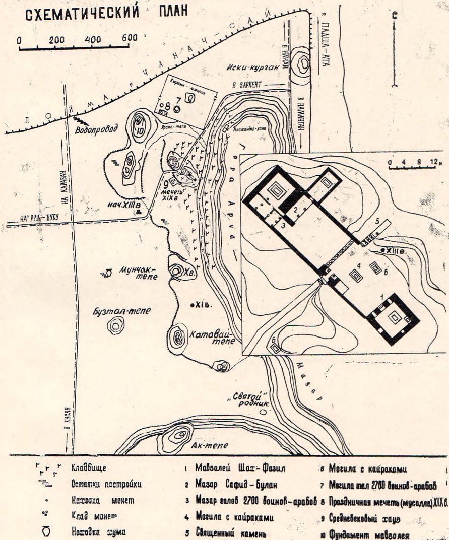
Рис. 36. Схематический план развалин средневекового Сафид-Булана.
