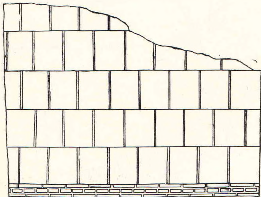
«Объект I. Характер пахсовых и сырцовых кладок стен замка. Внутренняя стена с полуциркульной аркой.
