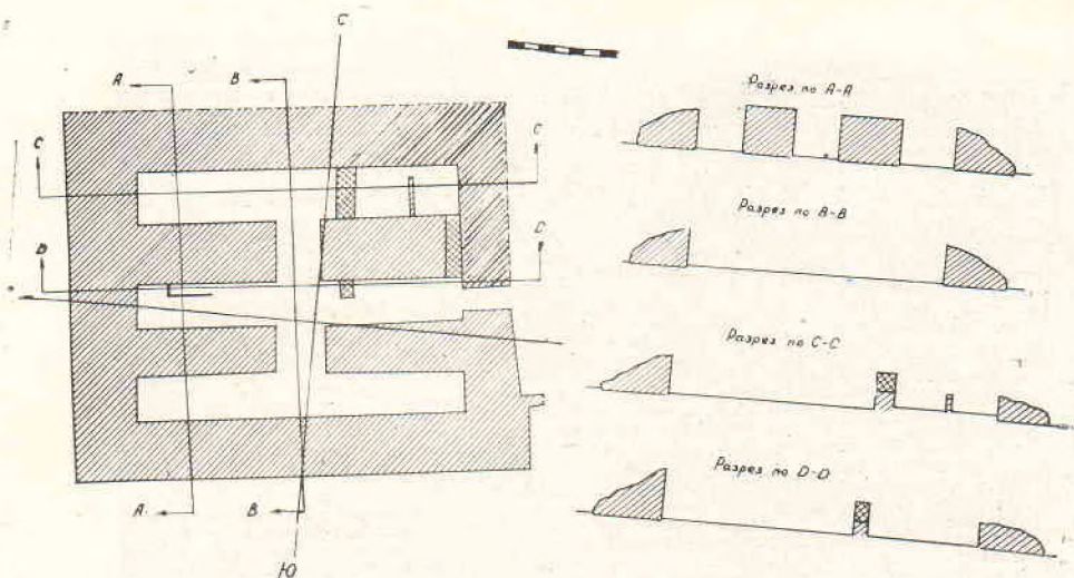
План и разрезы замкового сооружения (объект VII). Раскопки 1963 г.
