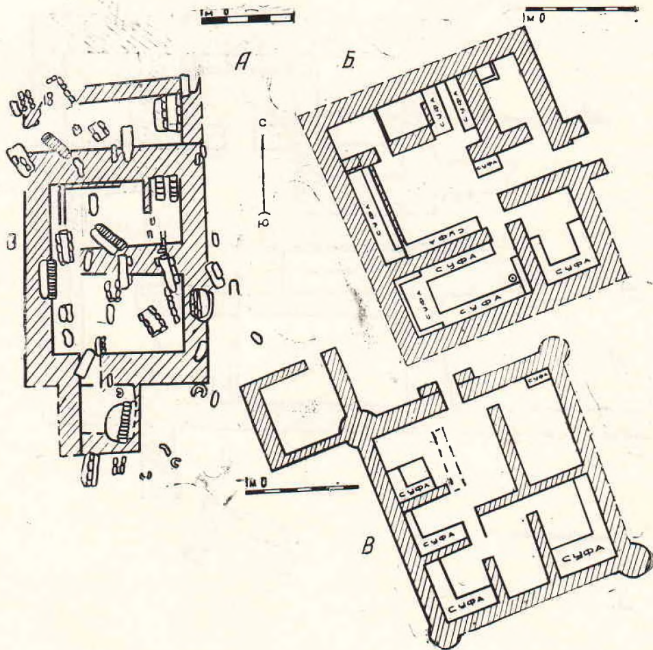
План жилого дома № 3 (объект VIII).
