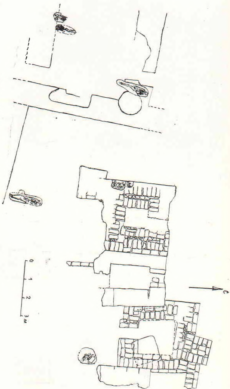
Раскоп II. Некрополь. План южной части раскопа на отметке 1,5 м. 1983 г.
