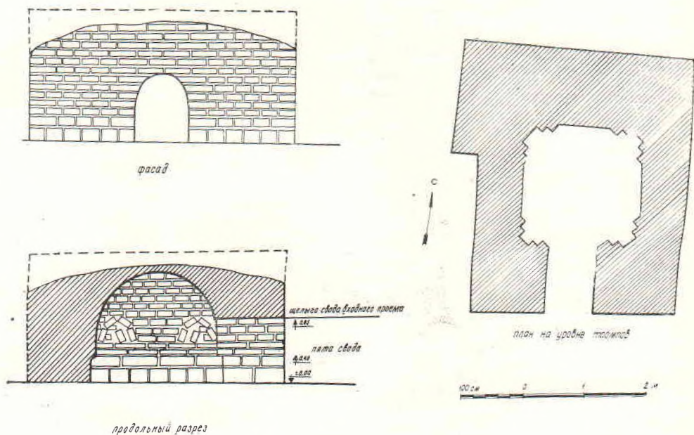
Наус № 4. План и разрез.
