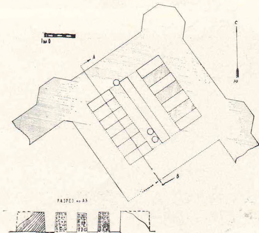
План замкового сооружения. Объект I. Третий строительный горизонт.
