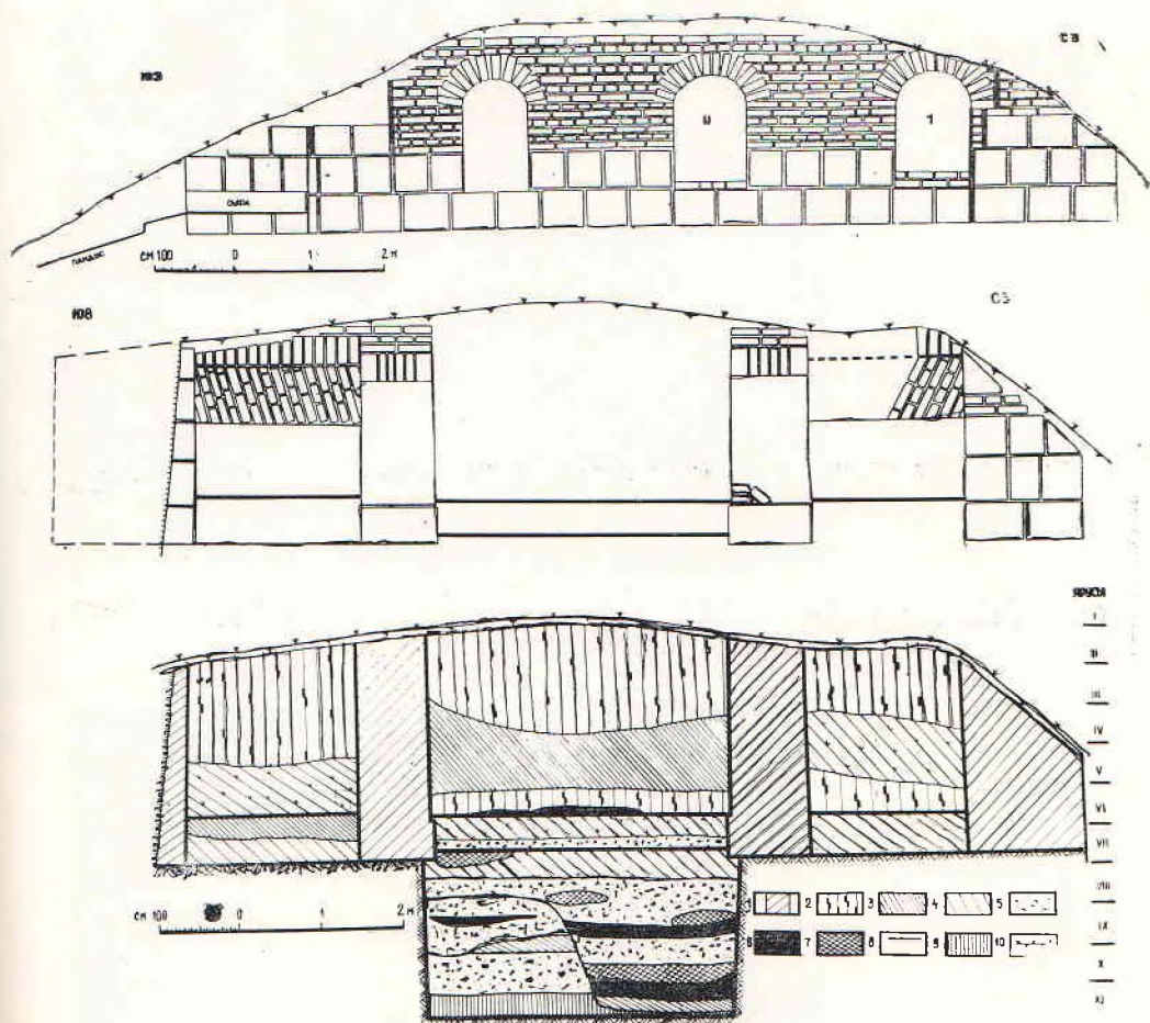
Раскоп IV. Архитектурный и археологический разрезы многокамерного науса. Раскопки 1978 г.
