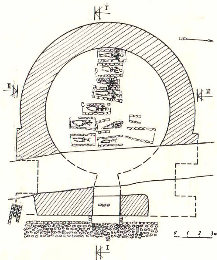
Рис. 12. План мавзолея № 2 (на уровне погребений).
