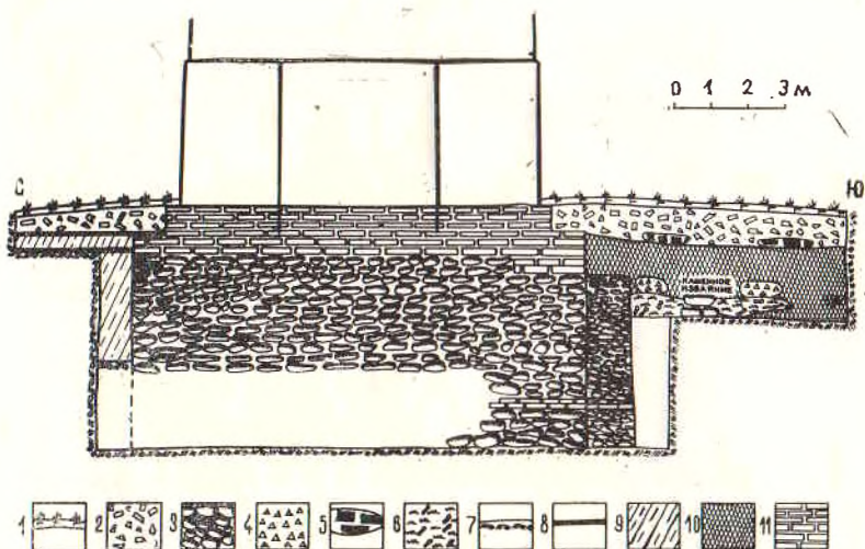
Рис. 8. Минарет. Разрез по основанию: 1 — дерновый слой; 2 — завал жженного кирпича; 3 — каменная кладка; 4 — скопление керамики; 5 — дерево; 6 — зола с косточками животных; 7 — материк; 8 — уровень пола; 9 — рыхлый слой глины; 10 — плотный слой глины; 11 — кирпичная кладка.
