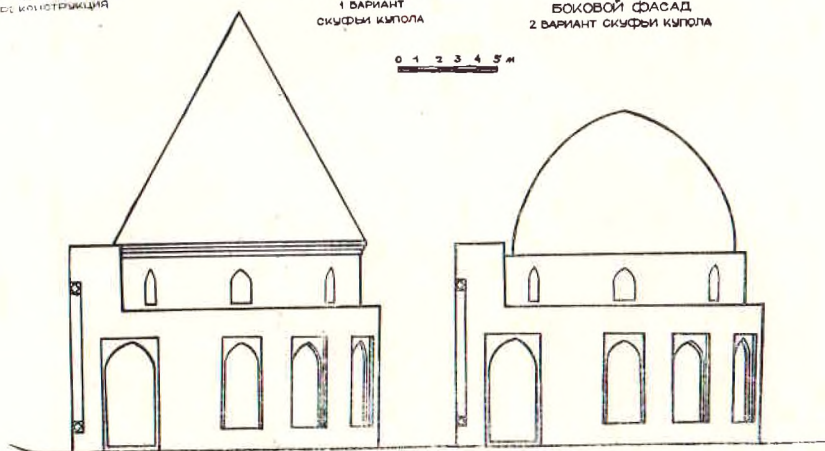
Рис. 15. Варианты реконструкции мавзолея № 2 (по Г. А. Пулаченковой)
