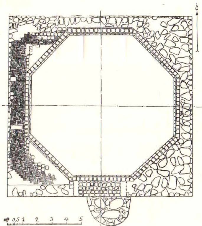
Рис. 7. План основания минарета, Раскопки 1970 г.
