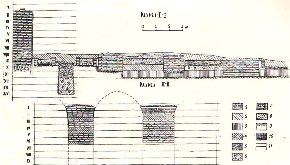
Рис. 19. Стратиграфический разрез раскопа в усадьбе: 1 — сырцовая кладка стен; 2 — рыхлый завал глины; 3 — уплотненный слой; 4 — пахса; 5 — плотный слой завала; 6 — завал кирпича, глины, керамики; 7 — каменная забутовка; 8 — песок; 9 — слой гальки; 10 — зола с углями; 11 — уровень пола.
