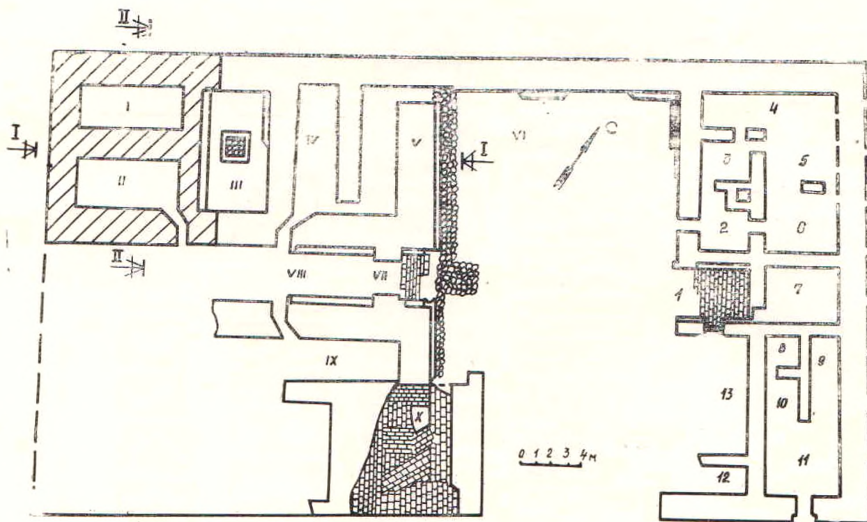
Рис. 18. План усадьбы в юго-восточном секторе городища. Раскопки 1972—1974 гг.
