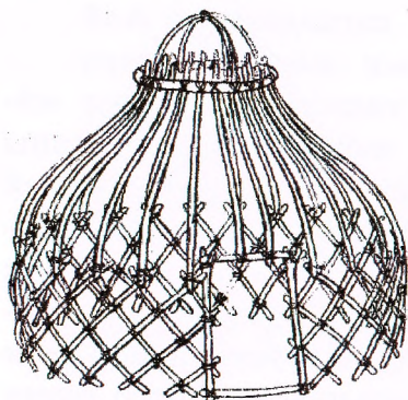
6-сүрөт. Алгачкы боз үйдүн соңкусу
