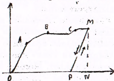
№1 диаграмма Механикалык күчтөн нерсенин деформацияланышынын көз карандылык диаграммасы. Мында: OA – серпилгич деформация; B – агуу чеги; BC – агуу аянтчасы; MP – күч-аракеттин токтолушу.
