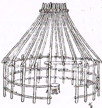
5-сүрөт. Алгачкы боз үй
