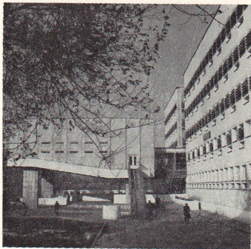
Институт русского языка и литературы по проспекту Мира в городе Фрунзе. Проект (архит. У. Алымкулов — руководитель, О. Лазарев, С. Султанов, Д. Аманалиев, Ж. Жанаалиев, инж. Л. Сидоренко, Е. Волошина и др.). 1985.
