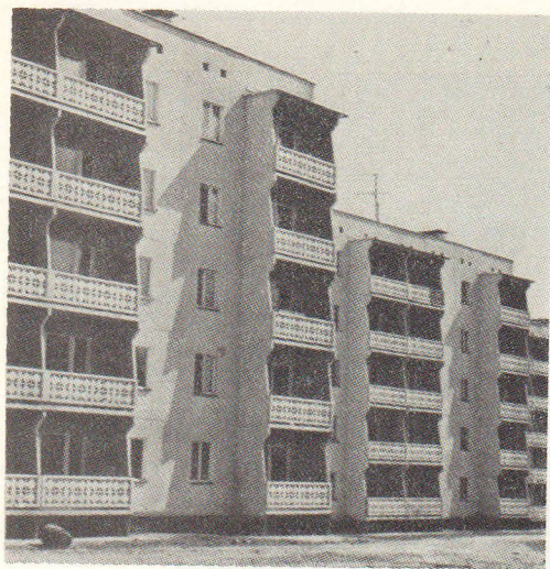
5-, 9-этажные жилые дома серии «105» в 9а микрорайоне в городе Фрунзе (архит. Е. Писарской, В. Седов, инж. В. Анистратов, А. Мозговой, А. Афонин, В. Тэвс). 1980.
