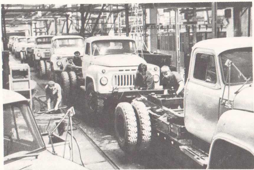
Главный конвейер производственного объединения «Киргизавтомаш».
