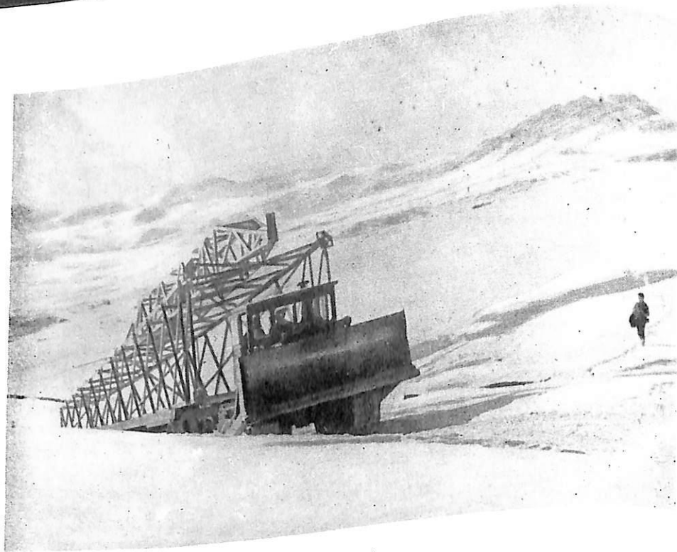
Тянь-Шандагы ЛЭП, Кум-Бел ашуусу (3600 м.)
