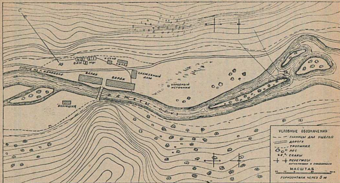
План курорта Джеты-Оуз (из статьи Н. М. Прокопенко „Термальные источники Тянь-Шаня“).
